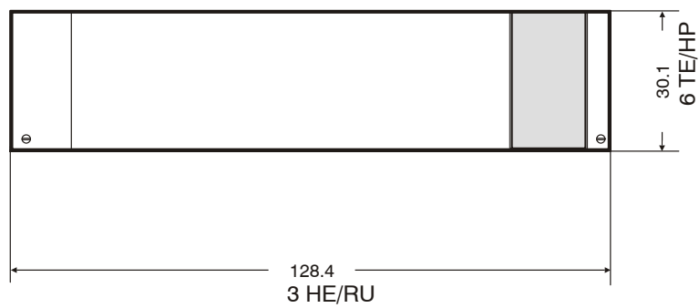
Dimensions A6151 Abmessungen A6151
